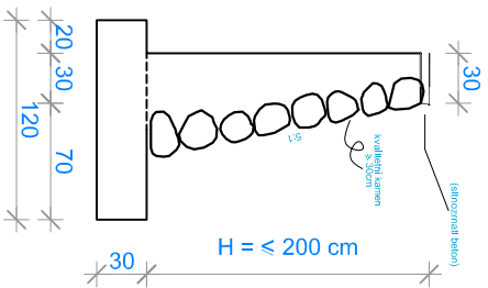
ARM. BET ZID OBLOŽEN KAMENOM Z3 TIP 3
